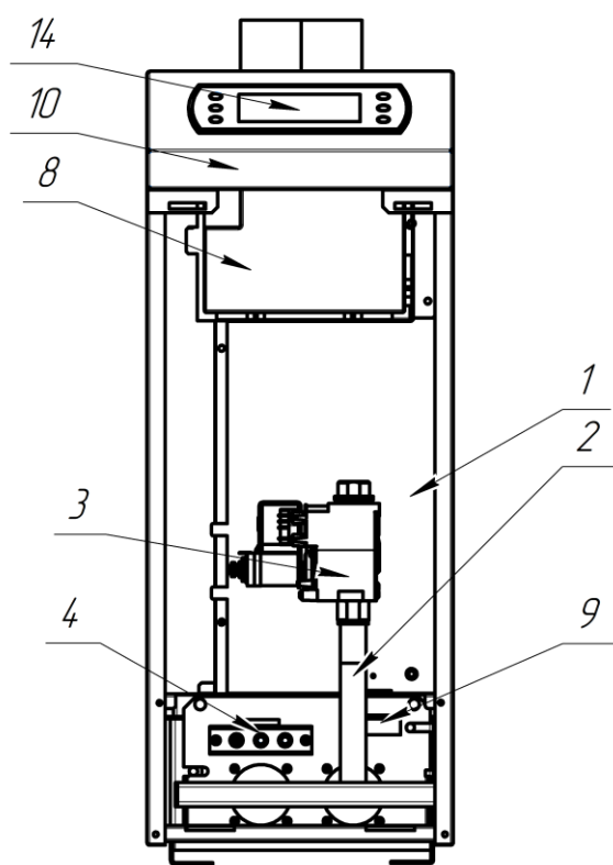
Рисунок 1 – Конструкция котла КОВ-СК(В)Се
